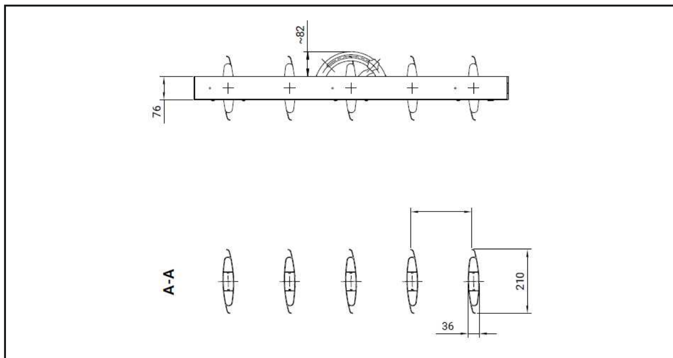
Obr. 2 : Schéma pozic vodící lišty slunolamu, pohonné páky a pozice jednotlivých lamel.
