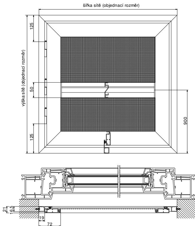
Obr.11 Schema vyměření sítě
